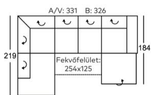
945-65, 200-126-DL, 846-65-B (946-65, 200-126-DL, 845-65-B)
